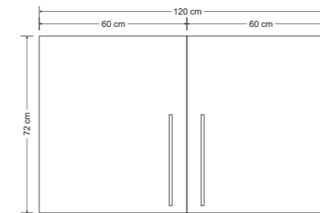
HS 120 - Skizze
